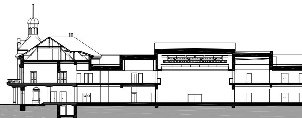
Příčný řez sálem 1:500
