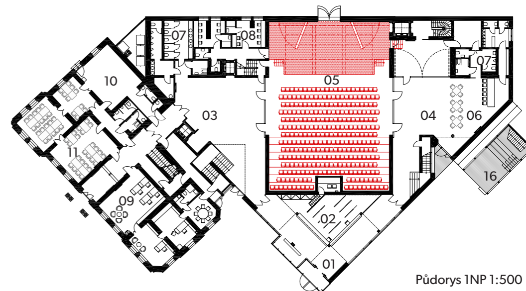
Půdorys 2NP 1:500
